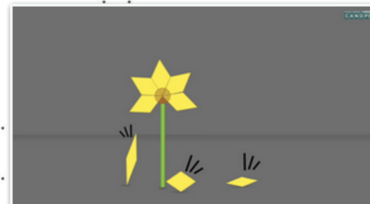
Axes de symétrie et diagonales du losange
